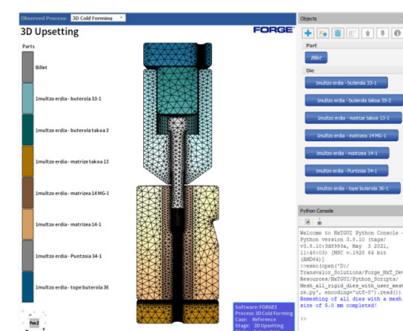
Exécution des scripts Multi_STL_files_loading.py et Mesh_all_rigid_dies_with_user_meshsize.py qui permettent d'obtenir ce résultat en quelques secondes seulement.
